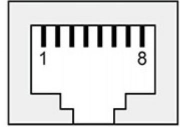
Abbildung 1: ttyS3 Pinout
